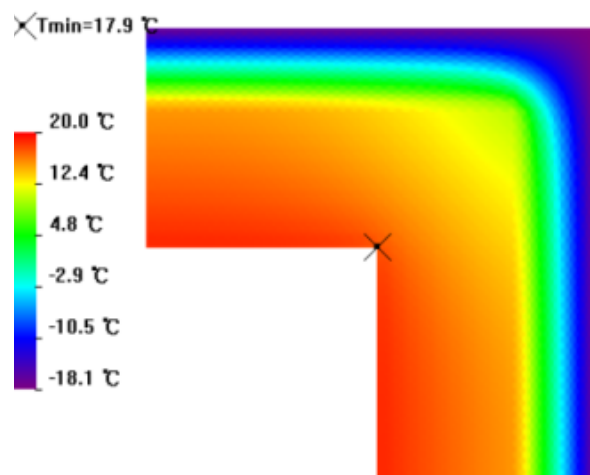
外墙阴阳角部位结露计算
