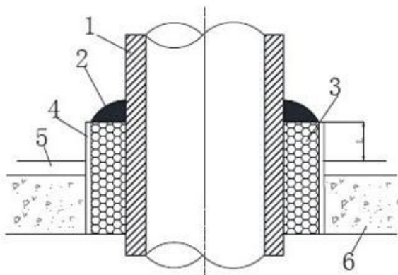
孔洞应采取密封隔声措施
