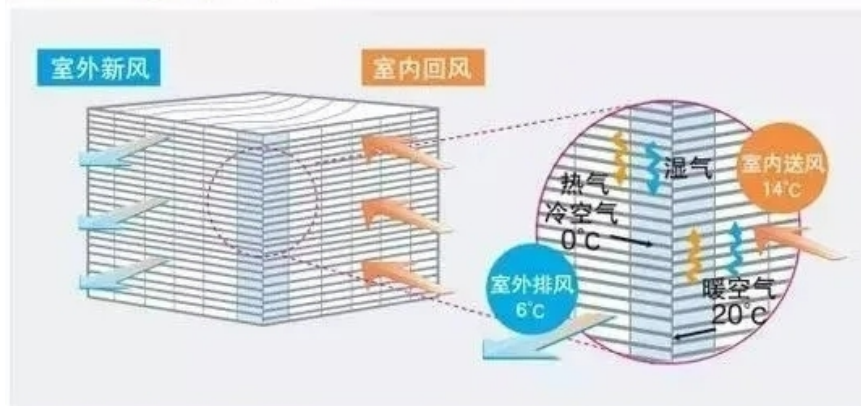
热交换芯内部(示意图)
