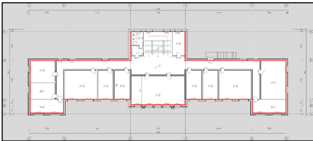
连续气密层示意图（平面）
