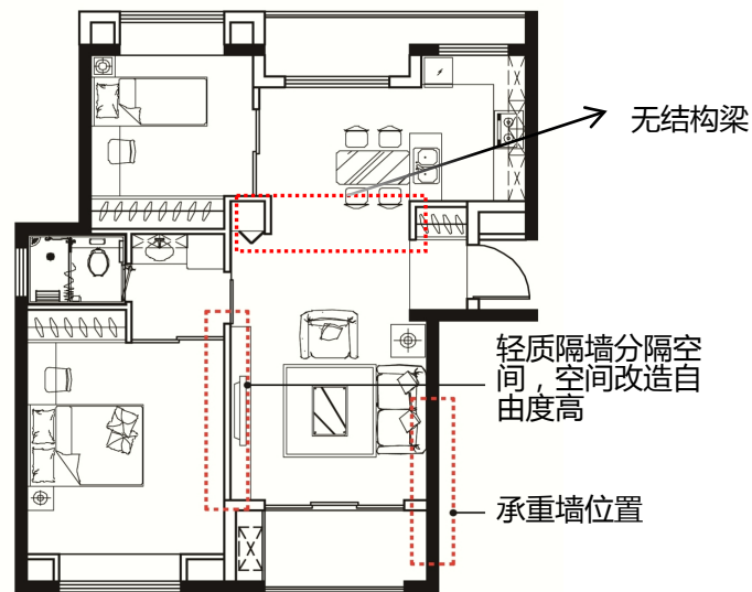
大空间结构平面设计
