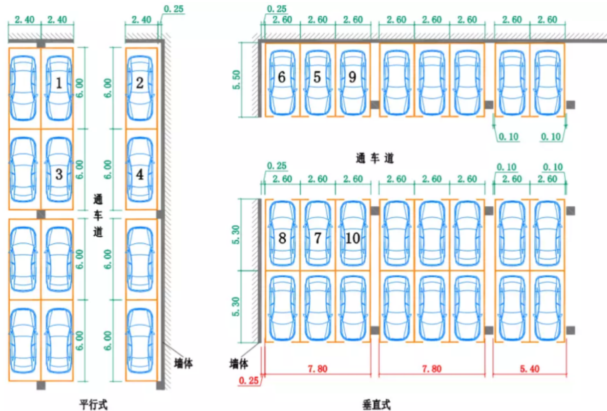
常见停车位示意图及建议尺寸（单位：m）——左：平行式、右：垂直式
