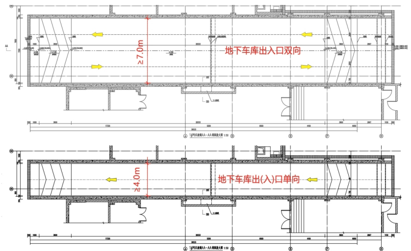
直线式单双车道净宽
