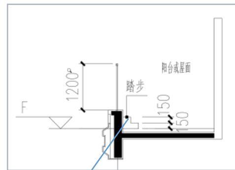
可登踏面起算安全高度
