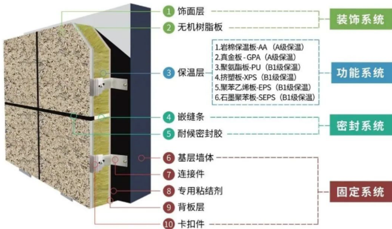
保温与结构一体化外墙技术
