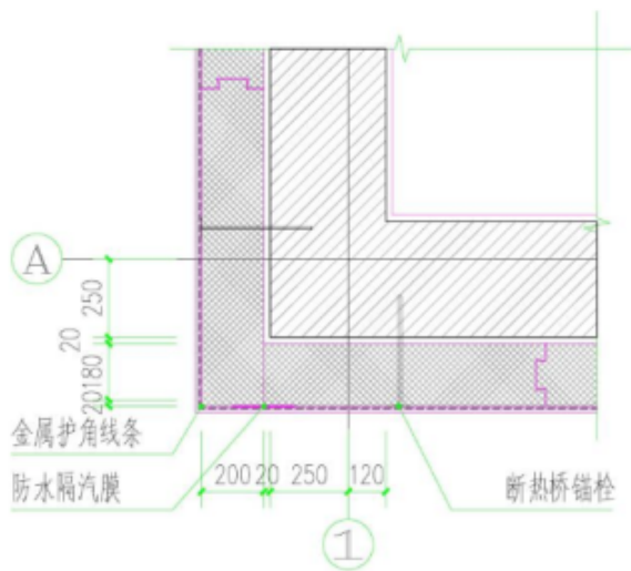
外墙整体热桥处理（阴阳角部位）
