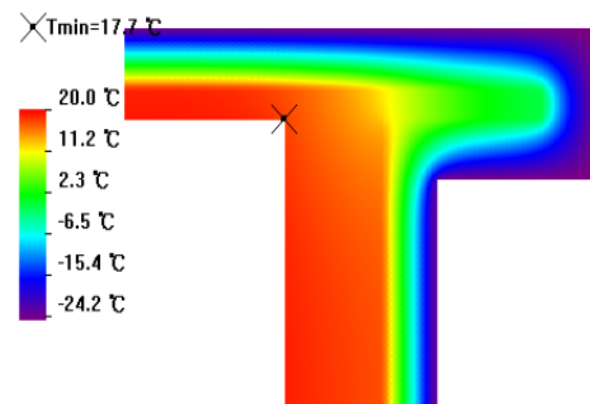
檐口部位结露计算
