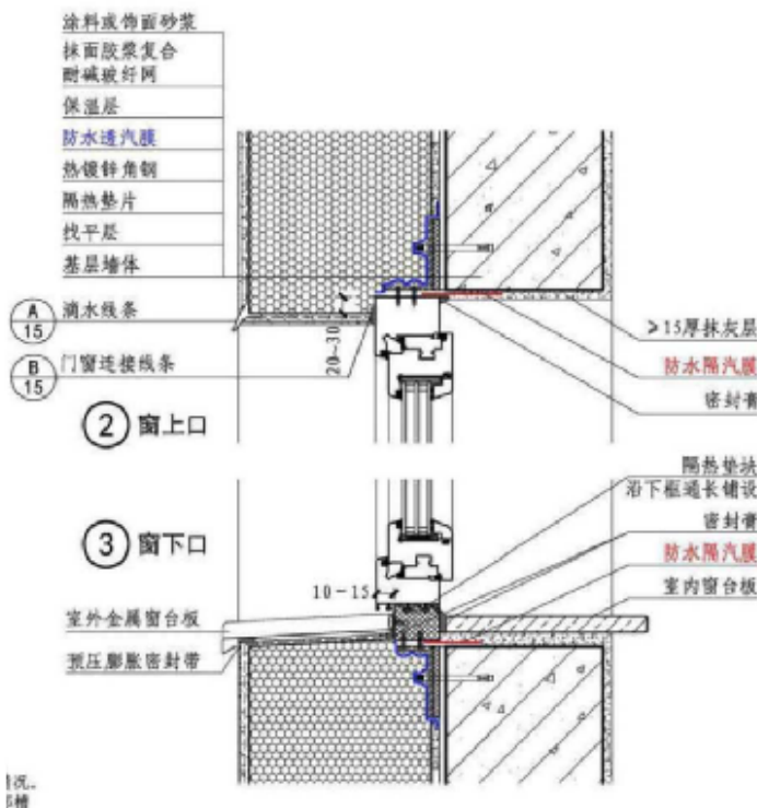
节能副框做法
