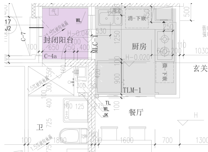
服务阳台
