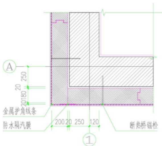
外墙整体热桥处理（阴阳角部位）
