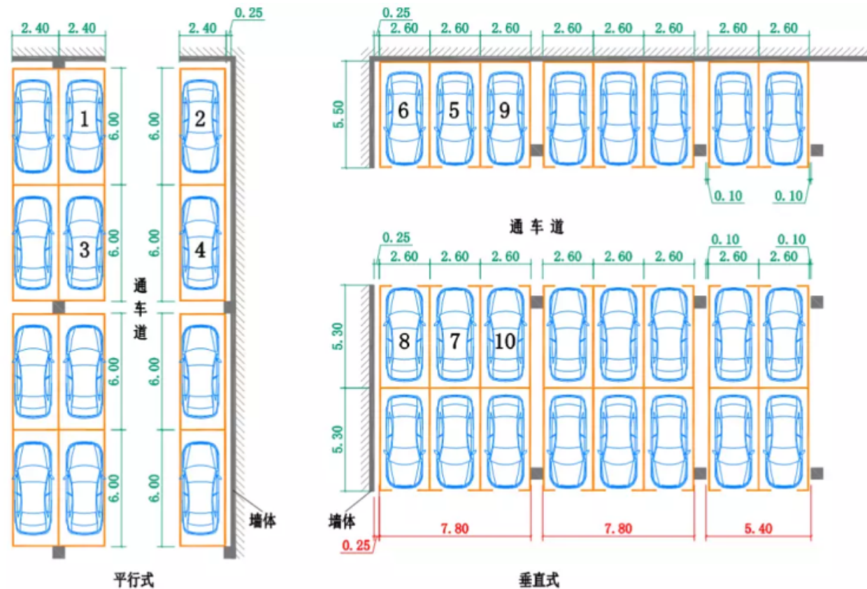
常见停车位示意图及建议尺寸（单位：m）——左：平行式、右：垂直式 本图所绘停车线线宽为10cm，可以看到停车线与小型汽车（4.8米*1.86米）车辆外廓、后视镜的位置关系
