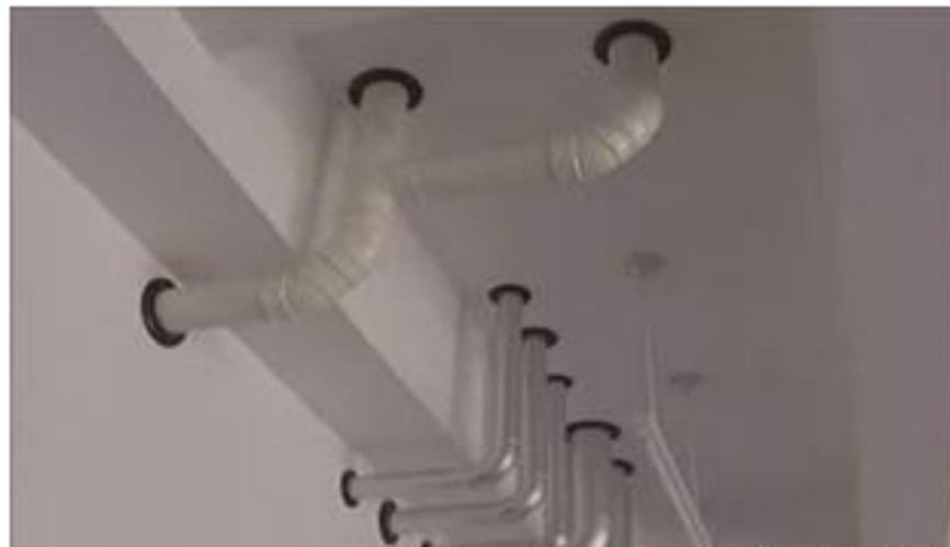
孔洞应采取密封隔声措施示例图
